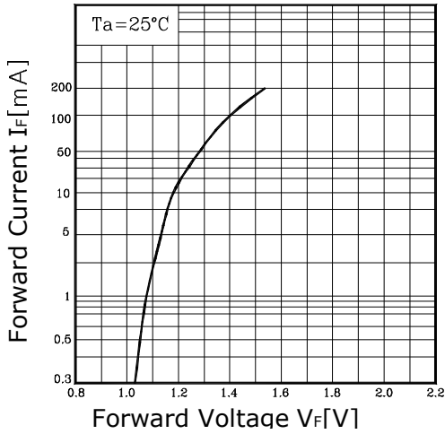
Fig.1 I_F - V_F
