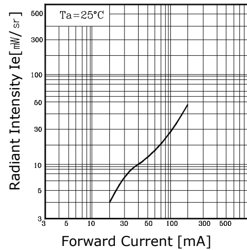
Fig.4 I_v - I_F
